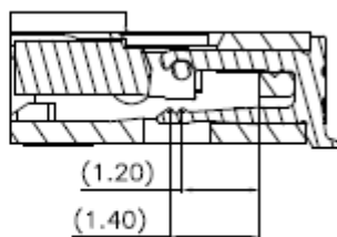
DETAIL A-A SCALE 2:1
