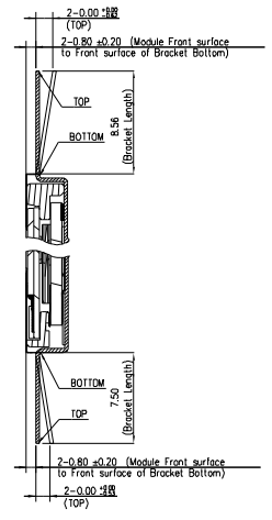
SECTION YY-YY SCALE 5:1
